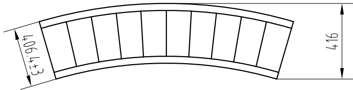
Максимально допустимое отклонение изгиба 最大允许弯曲公差
